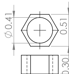
Nut
